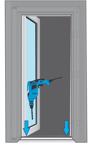
Etape 8. Fixez la coulisse dans le plancher avec 2 chevilles
