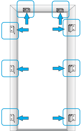
Etape 1. Fixez les pinces sur le dormant.
