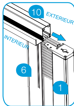
Etape 6b. Clipsez la coulisse sur la partie saillant du couvercle du coffre
