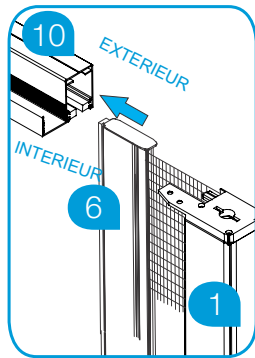
Etape 6a. Introduisez la bare de tirage a l'interieur de la coulisse laterale
