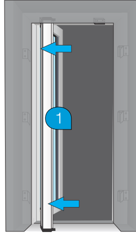
Etape 3. Introduisez le coffre dans l'espace prevue pour le montage
