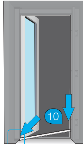
Etape 7. Montez la coulisse inferieure en repetant les etapes 6a et 6b
