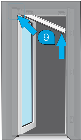
Etape 6. Montez la coulisse superieure en faisant en meme temps les etapes
